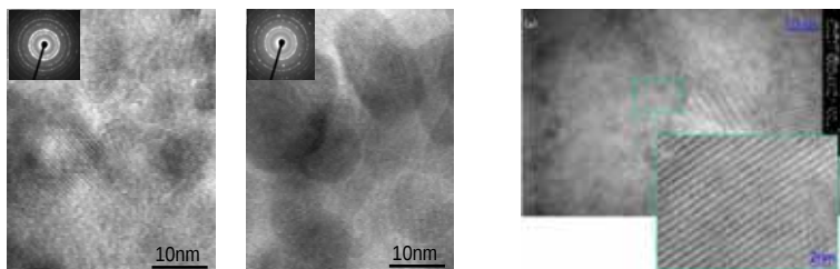
CaMg-V, CaMg-Fe系合金の格子像・回折像
