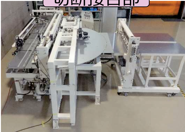
切断接合部
