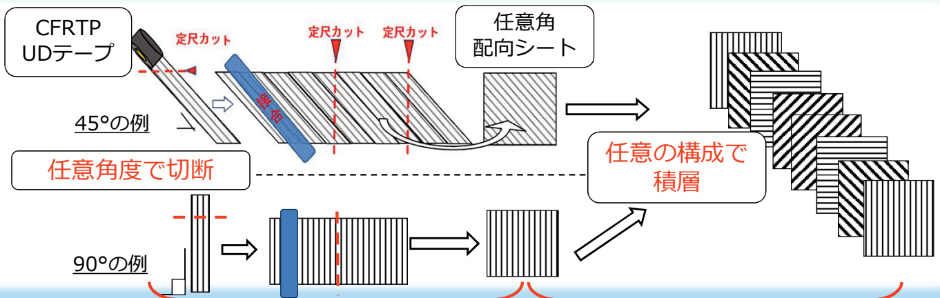
切断接合部
