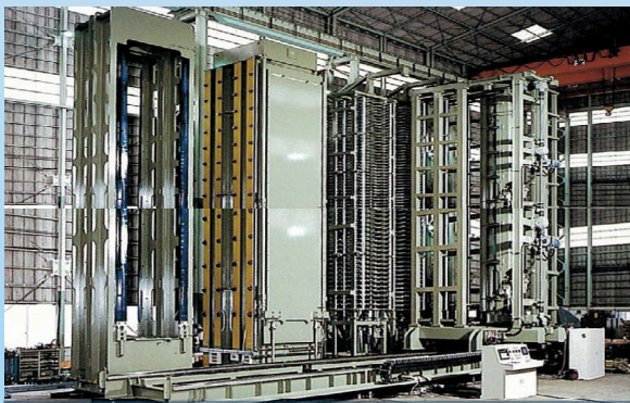
銅張積層板成形用36段真空プレス
